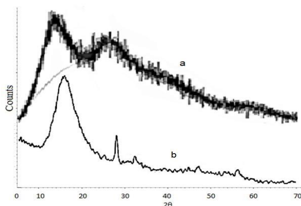
Рис. 5. Дифрактограммы поли-N-винилпирролидона (а) и комплекса Pd 0 -поли-N-винилпирролидон (б).
